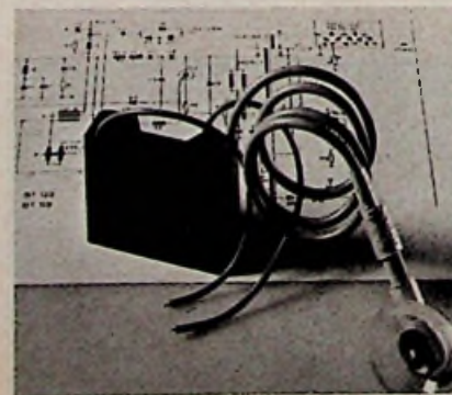
Bild 5: Neue 25-kV-Hochspannungskaskade TM 25-20 in Siliziumtechnik (ITT Bauelemente)
