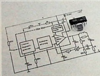
Bild 3: Integrierte Bildklippschaltung TDA 1044 (Intermetall)
