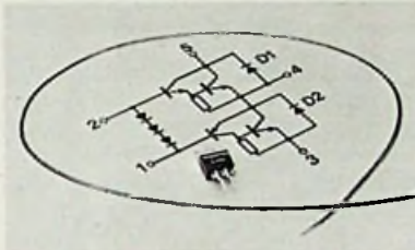
Bild 7: Monolithischer Dual-Komplementär-Darlington L 142 (SGS/Ates)
