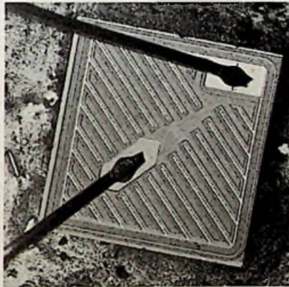
Bild 8: Chip des epitaxialen NPN-Silizium-Transistors BU 406 / BU 407 für Horizontalablenk-Endstufen (SGS/Ates)
