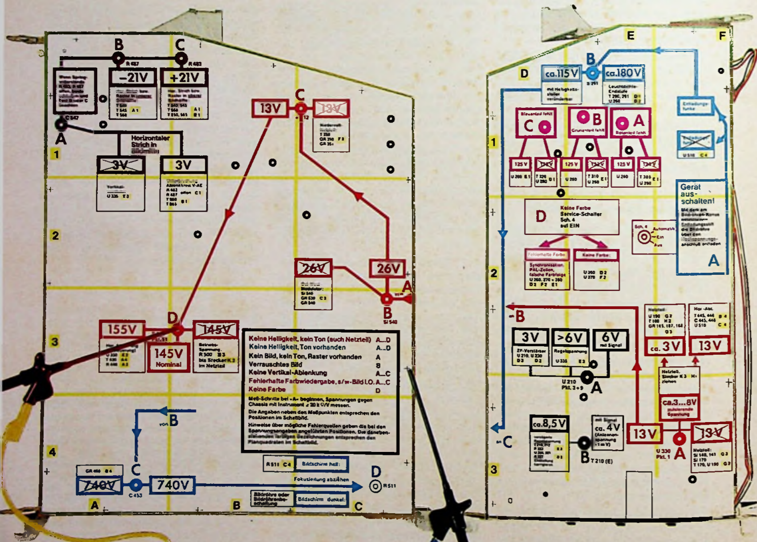
Transparente Diagnose-Schablonen für Großsignal- und Kleinsignalplatte.
