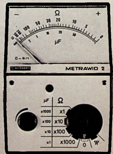
Widerstands-Kapazitäts-Meßgerät „Metrawid-2“ (Metrawatt)
