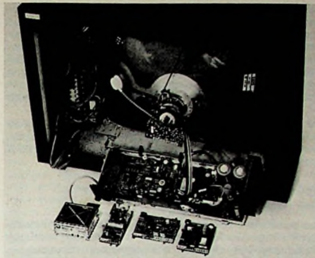
Bild 1. In den neuen Modul-Chassis für Metz-Schwarz-Weiß-Fernsehempfänger sind die Modul-Steckkarten und sonstigen Baugruppen steckbar ausgeführt
