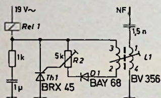
Bild 1: Teilschaltbild der thyristorgesteuerten Schaltstufe einer Ultraschall-Fernbedienung
