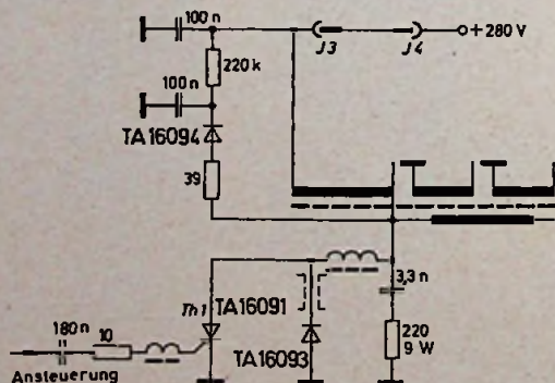
Bild 2: Teilschaltbild einer Thyristor-Zeilensablenkstufe mit Rücklaufthyristor
