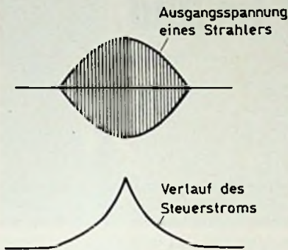
Bild 10: Zeitlicher Verlauf der Abtastströme
